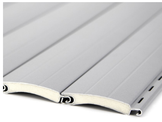
Aluminium-Profil CD 942
