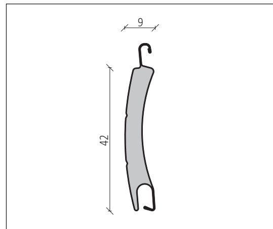
Aluminium-Profil CD 942
