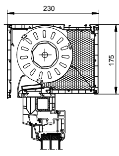
Tanext 175 Kasten 175 bis max. 1750 mm Elementhöhe
