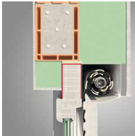
Möglichkeit 4: Fensterrahmendraufdoppelung eines Punext-Rollladens, Beispiel Putzmauerwerk/WDVS. Die Option der Rahmendraufdoppelung kann beim nachträglichen Einbau von Punext generell angewendet werden.
